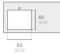
Hole size for the P1 sink Foratura top per vasca P1 Größe der Bohrungen für Beck P1
