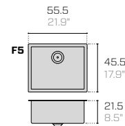
Satin overtop sink Vasca satinata sopratop Satiniertes Überbaubecken
